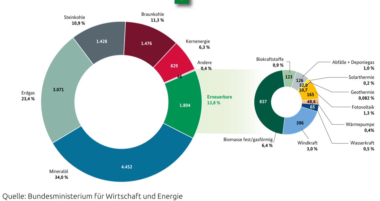
3. Primärenergieverbrauch in Deutschland 2018 (13.106 PJ*)
